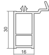
Арт. 142 Подставочный профиль: KBE 58 мм, PROPLEX, EXPROF, FUNKE, KRAUSS, NOVOTEX 58мм, VITRAGE 58 мм, GRAIN, GOODWIN 58 мм
