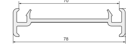
Арт. 350 Соединительный профиль: KBE 70 мм, VEKA 70 мм, TROCAL 70 мм, PROPLEX 70 мм, FUNKE 70 мм, KRAUSS 70 мм, NOVOTEX 70 мм, GRAIN 70 мм, VITRAGE 70 мм, GOODWIN 70 мм
