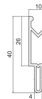
Арт. Т50-01 Термовставки ПВХ для фасадных систем СИАЛ "КП50", АЛЮТЕХ "ALT F50", KRAUSS "KRF-50", INICIAL "IF 50"
