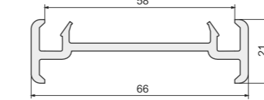
Арт. 150 Соединительный профиль: KBE 58 мм, VEKA 58 мм, PROPLEX 58 мм, EXPROF 58 мм, FUNKE 58 мм, KRAUSS 58 мм, NOVOTEX 58 мм, GRAIN 58 мм, VITRAGE 58 мм, GOODWIN 58 мм
