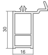
Арт. 142 Подставочный профиль: KBE 58 мм, PROPLEX, EXPROF, FUNKE, KRAUSS, NOVOTEX 58 мм, VITRAGE 58 мм, GRAIN, GOODWIN 58 мм
