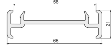
Арт. 150 Соединительный профиль: KBE 58 мм, VEKA 58 мм, PROPLEX 58 мм, EXPROF 58 мм, FUNKE 58 мм, KRAUSS 58 мм, NOVOTEX 58 мм, GRAIN 58 мм, VITRAGE 58 мм, GOODWIN 58 мм
