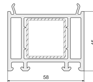
Арт. BP45 (арт. VEKA - 114.011) Расширитель: VEKA 58 мм, PLAFEN 58 мм Classic-line, RIGAP, OPAC
