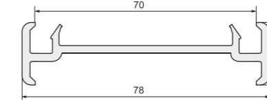
Арт. 350 Соединительный профиль: KBE 70 мм, VEKA 70 мм, TROCAL 70 мм, PROPLEX 70 мм, FUNKE 70 мм, KRAUSS 70 мм, NOVOTEX 70 мм, GRAIN 70 мм, VITRAGE 70 мм, GOODWIN 70 мм
